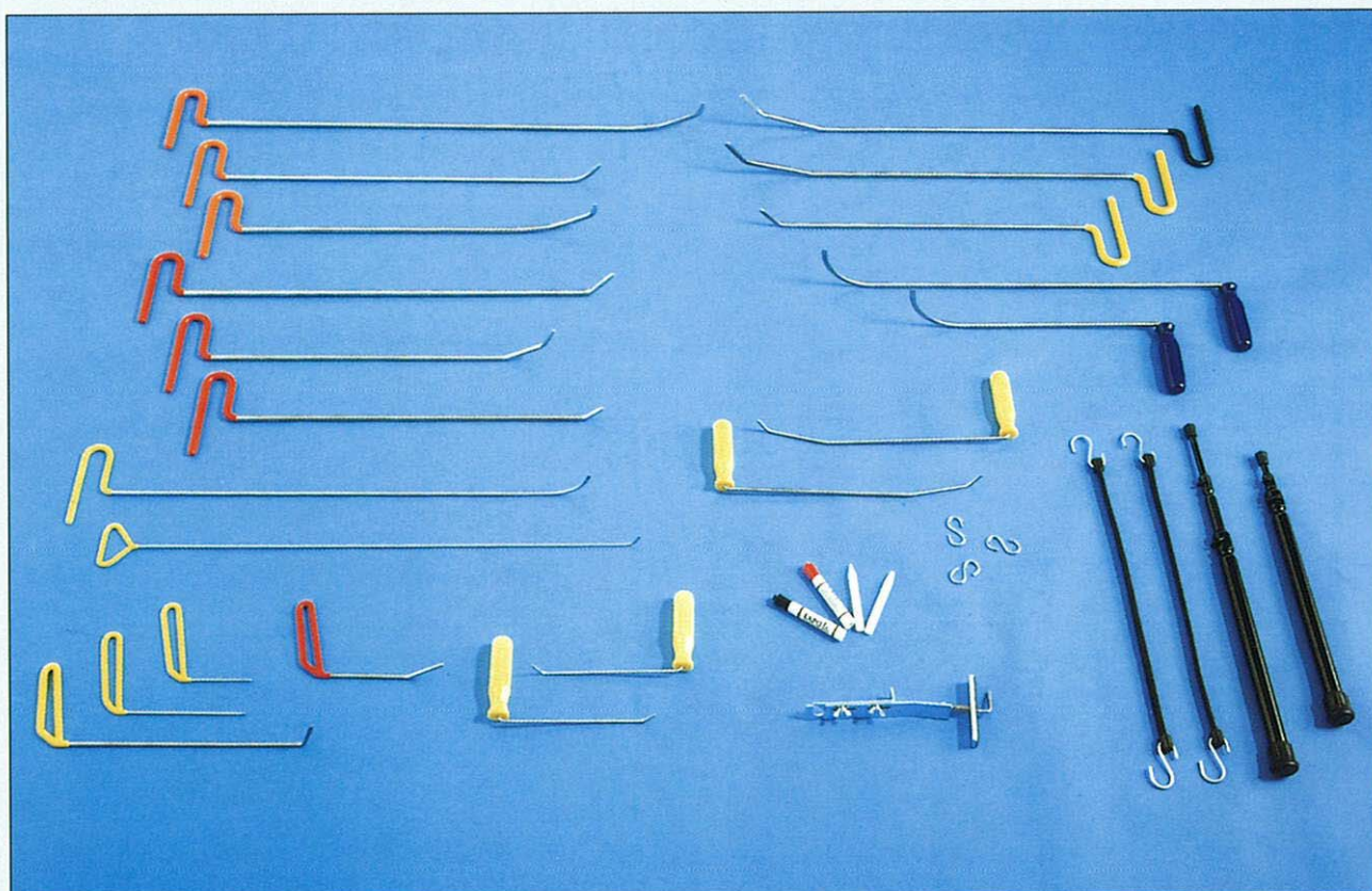
Custom kit met 21 gereedschappen (art.nr. 6526)
