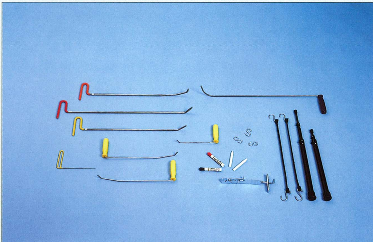
Starter kit met 8 gereedschappen (art.nr. 6512)
